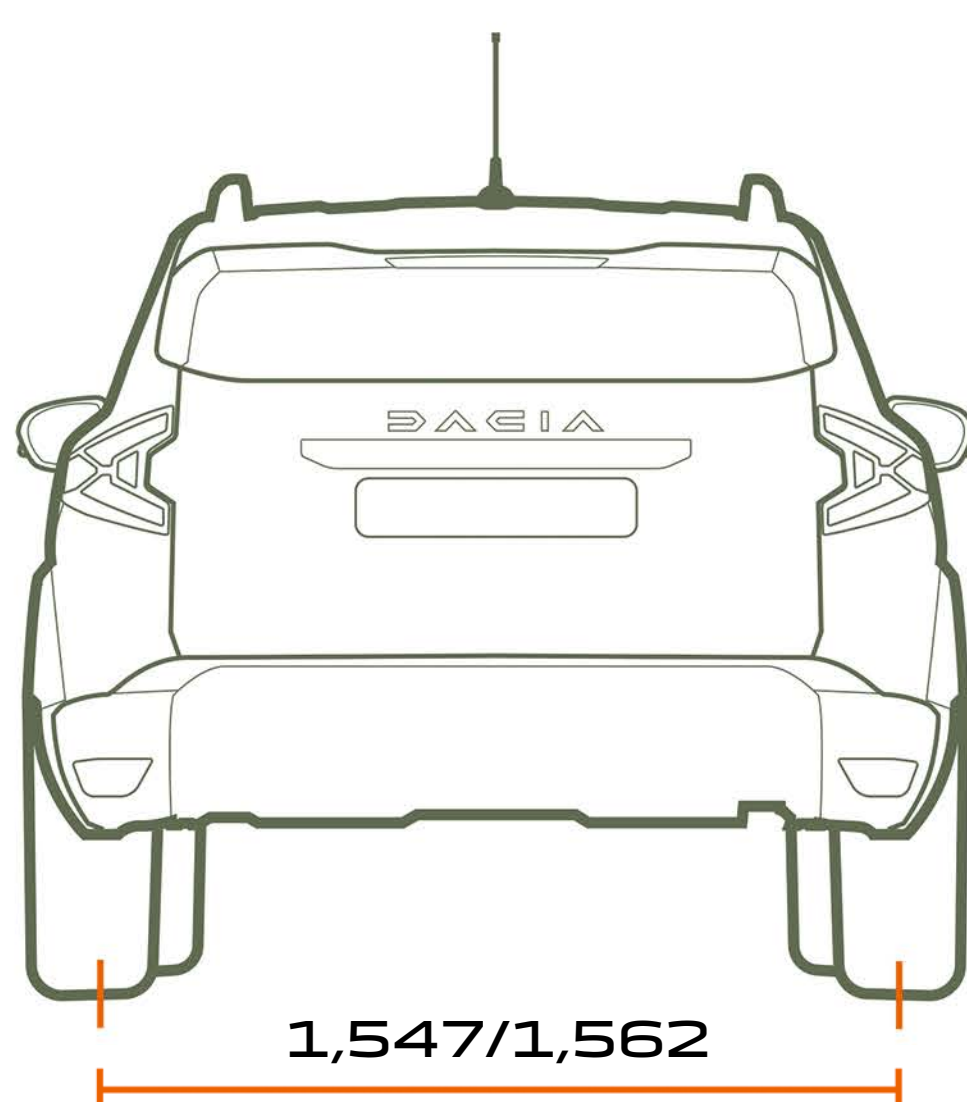
VISTA TRASEIRA
